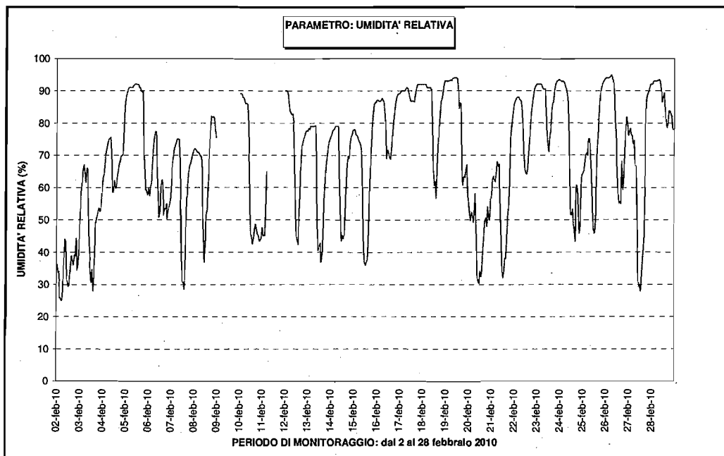
Figura 5: Umidità relativa
