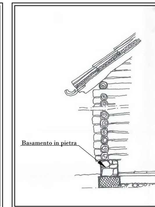
Schema strutturale
