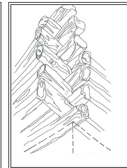
Schema incastro tra due pareti lignee
