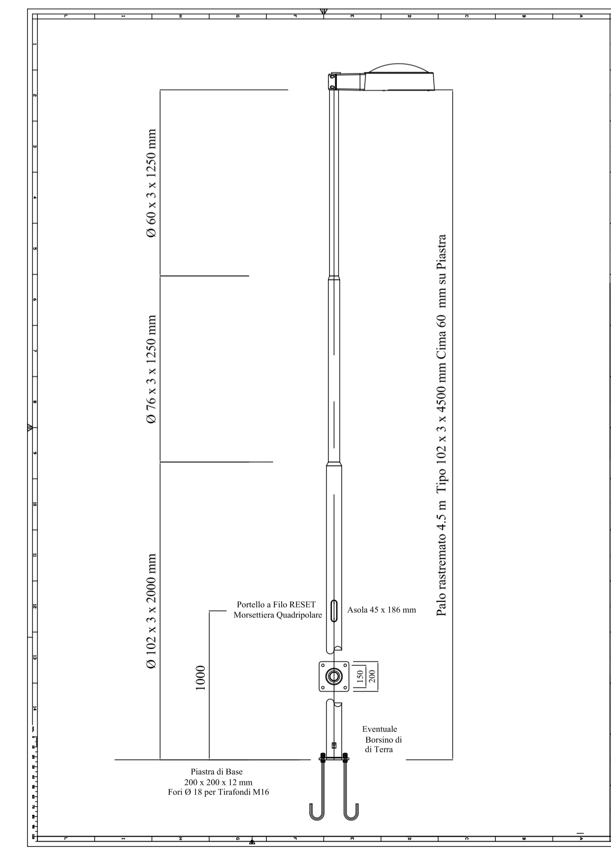
PARTICOLARE COSTRUTTIVO PALI ED APPARECCHI ILLUMINANTI - Scala 1:25 VERSIONE CON PIASTRA PER FISSAGGIO SU CORDOLO
