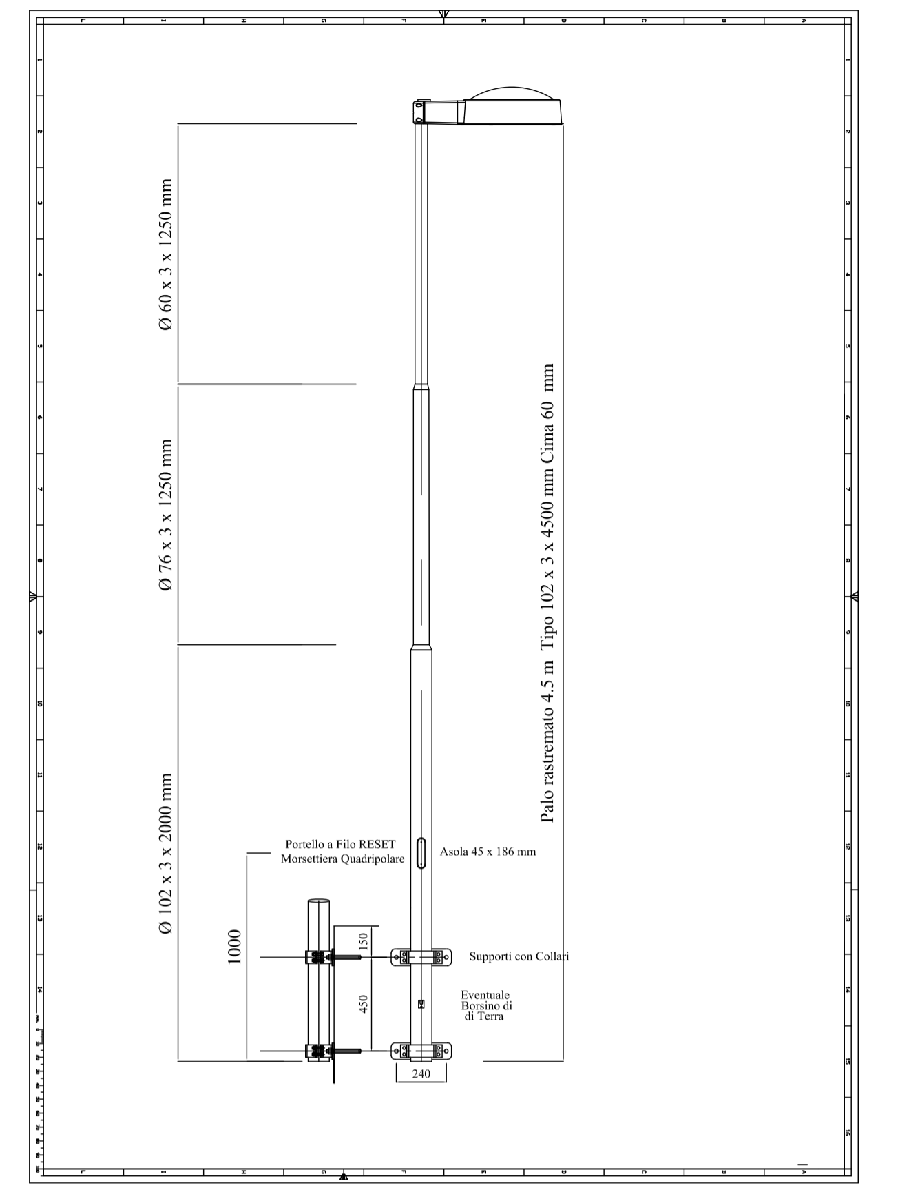
PARTICOLARE COSTRUTTIVO PALI ED APPARECCHI ILLUMINANTI - Scala 1:20 VERSIONE CON COLLARI PER FISSAGGIO SU MURO
