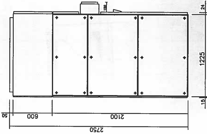
VISTA LATERALE
