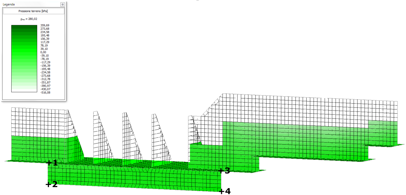
Figura 7-1 – Pressione sul terreno indotte dalle sovrastrutture derivanti dal modello di analisi strutturale e punti notevoli per l'individuazione delle pressioni del terreno.
