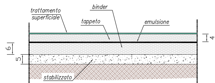
PARTICOLARE PAVIMENTAZIONE TRATTO
