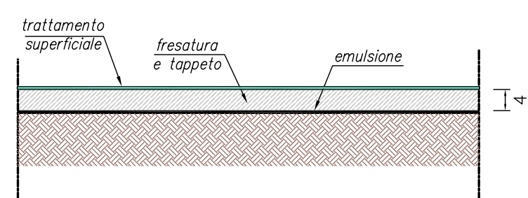
PARTICOLARE PAVIMENTAZIONE TRATTO
