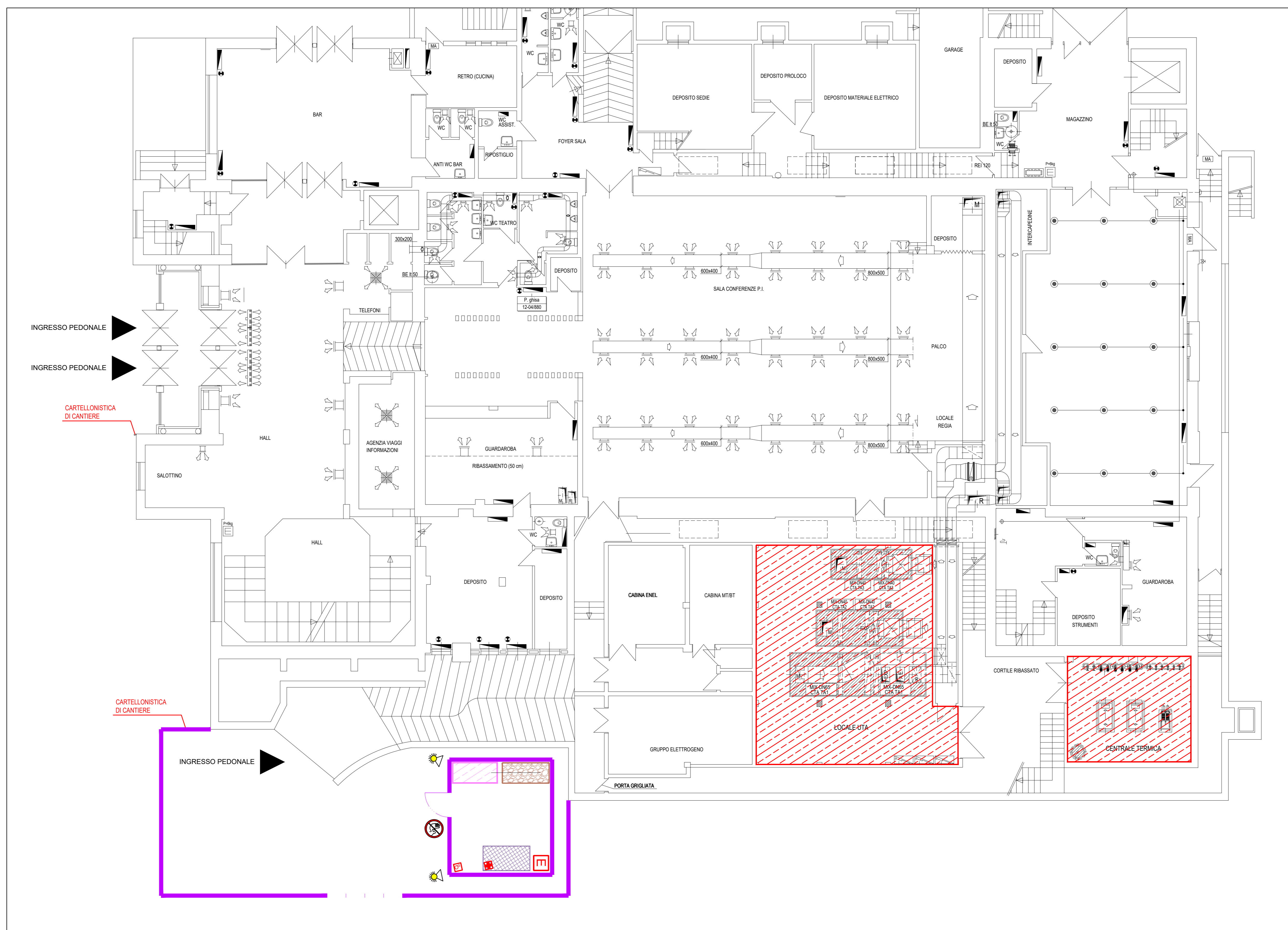
PLANIMETRIA PIANO TERRENO SCALA 1:200
